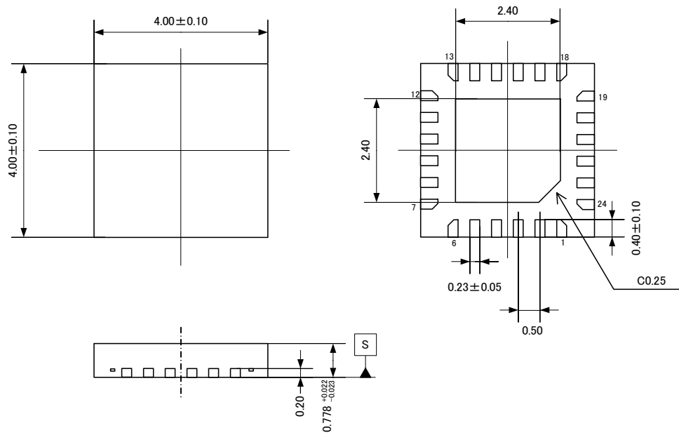
Fig. 15 Outer Dimensions
