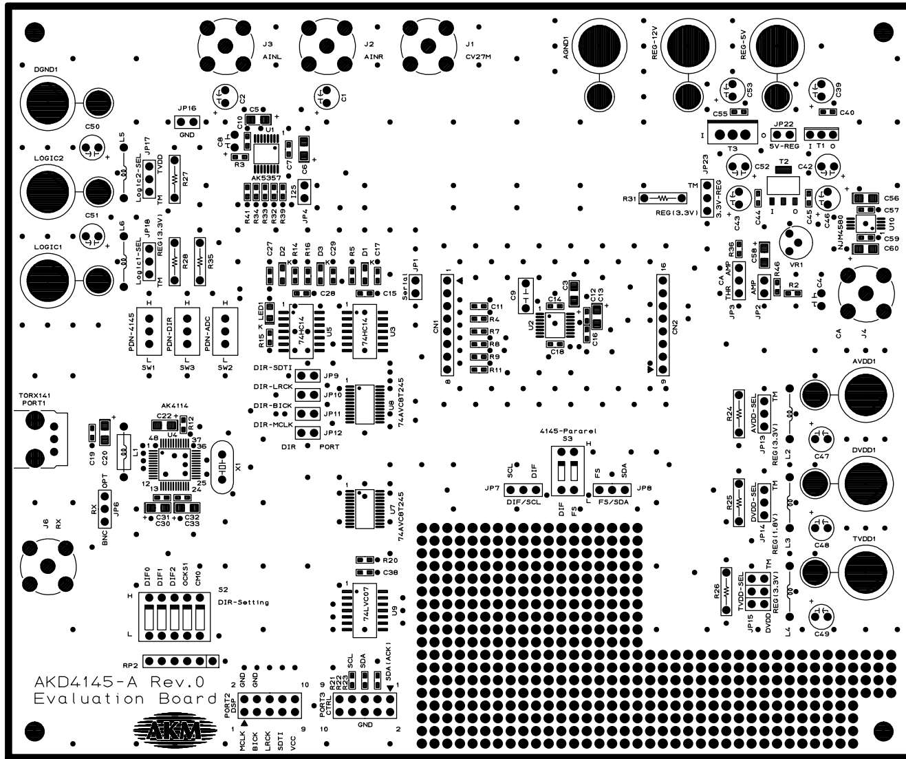
AKD4145-A L1 SILK
