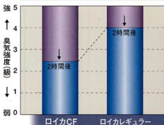
イソ吉草酸の消臭性能(※B)
