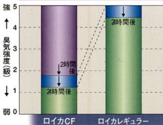
アンモニアの消臭性能(※A)
