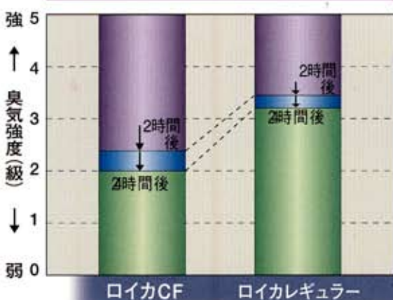
酢酸の消臭性能(※A)
