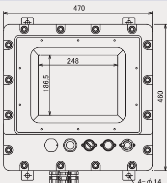
EXGP-3600R 外形図
