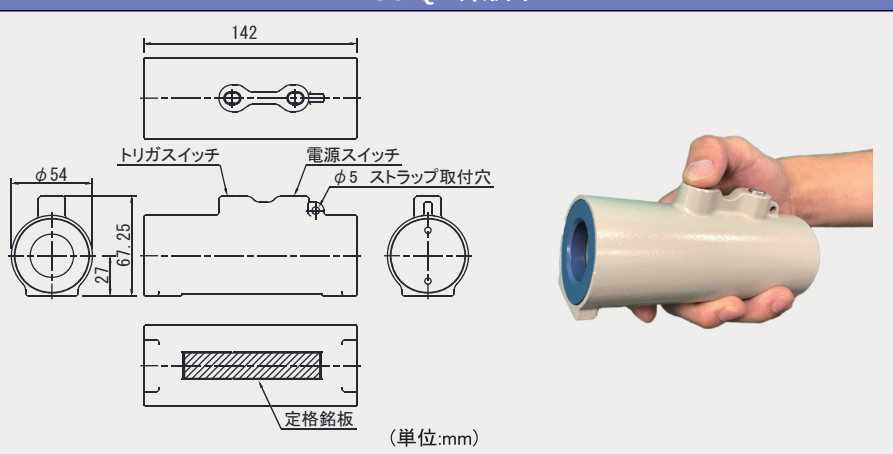
EXSC-QB 外形図
