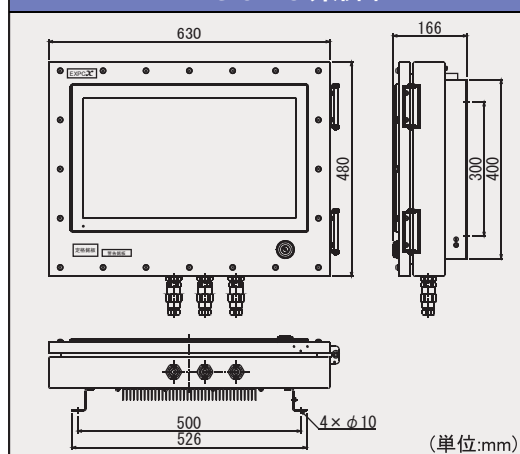
EXPC-6220 外形図
