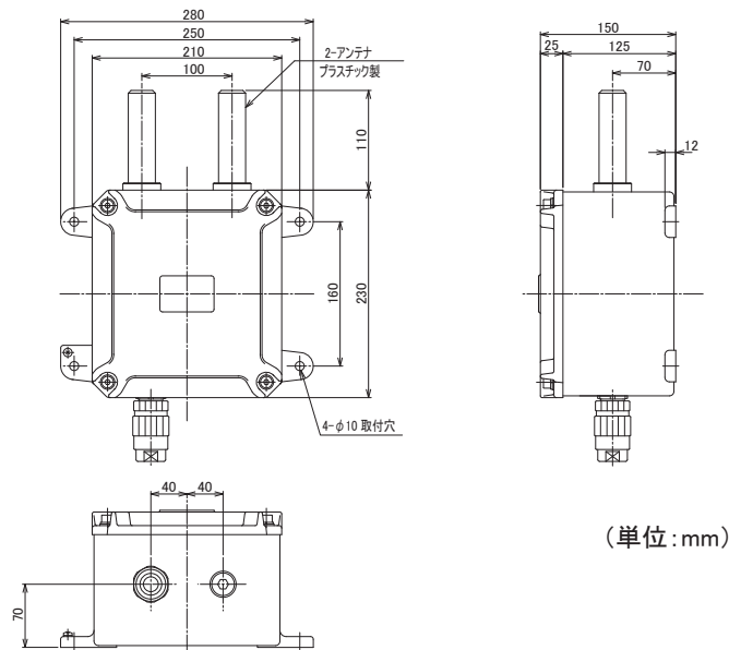
外形寸法
