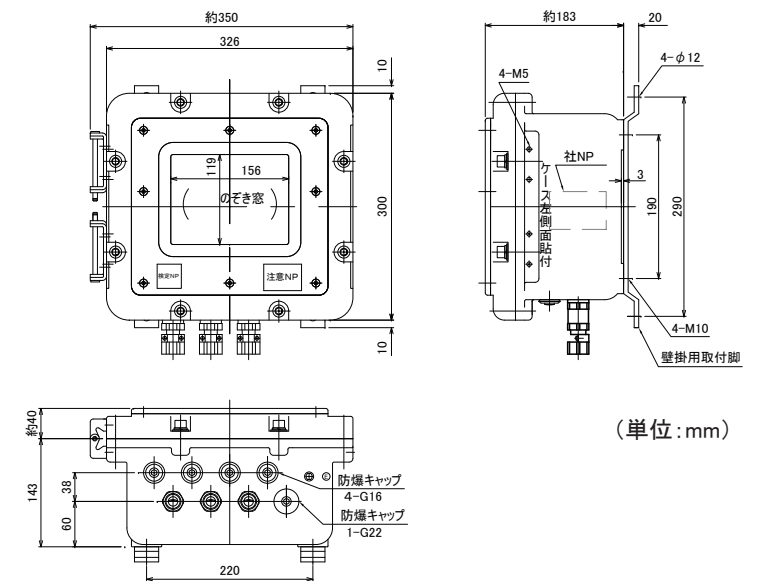
外形寸法
