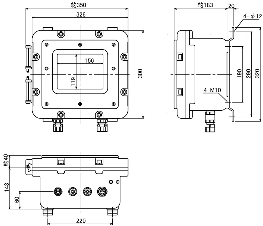
图 3-8 寸法图
