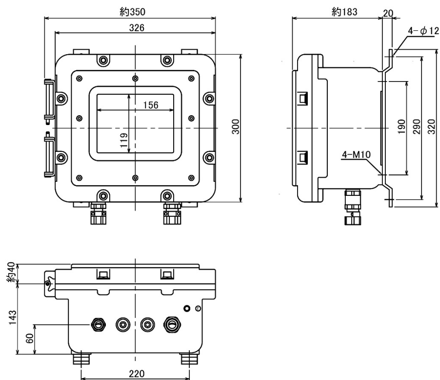
図 3-8 寸法図
