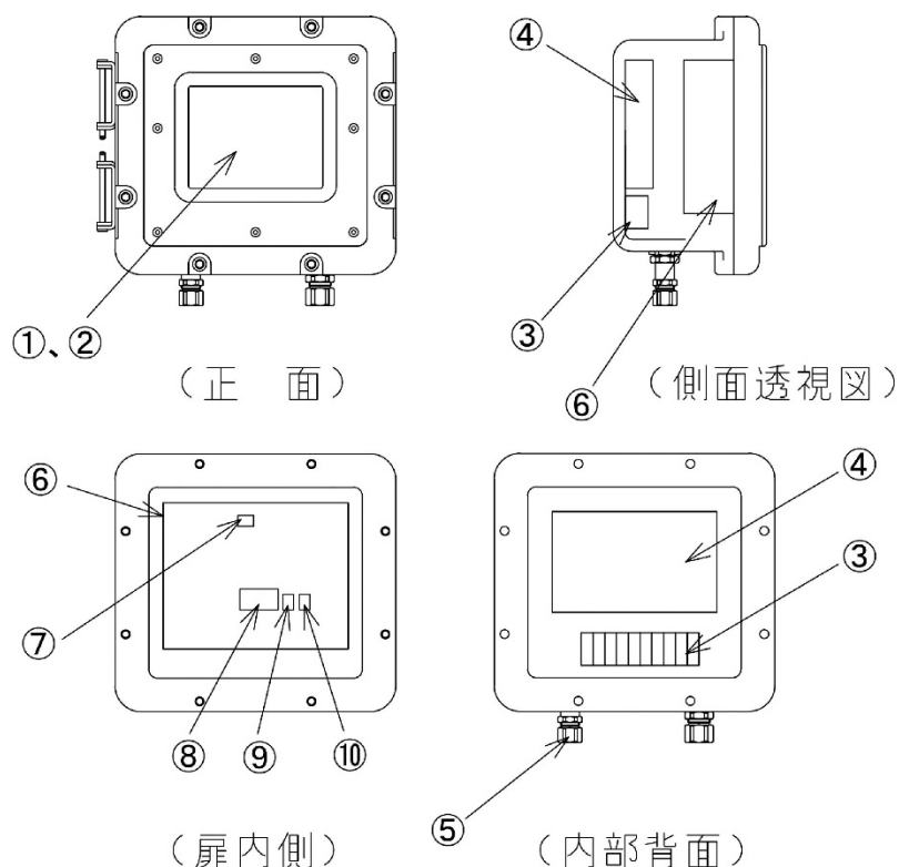
図 3-9 全体図
