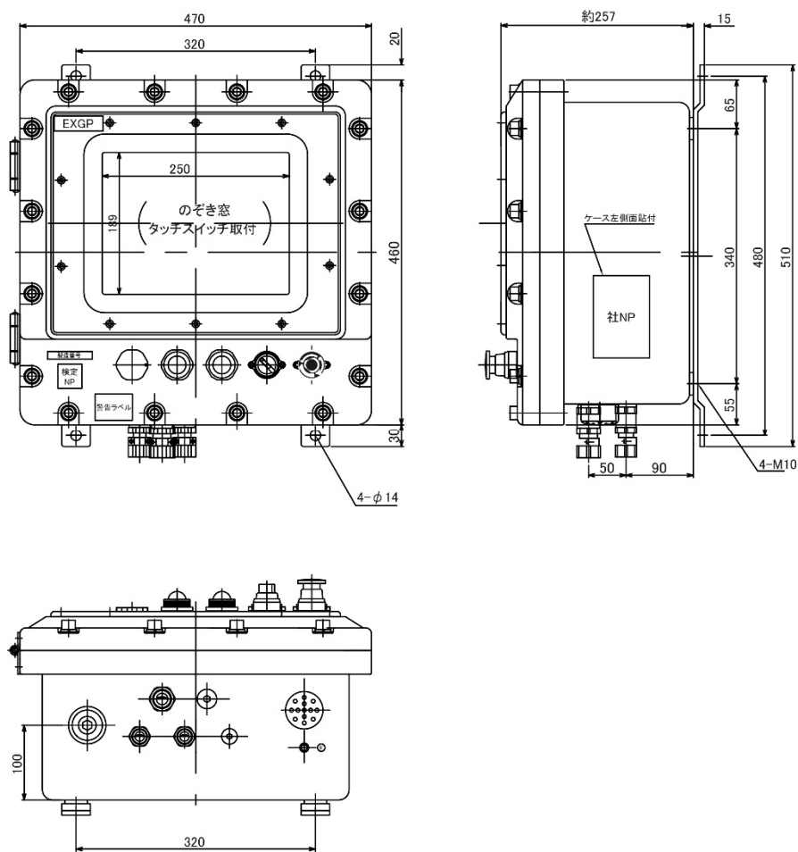
図 3-8 寸法図
