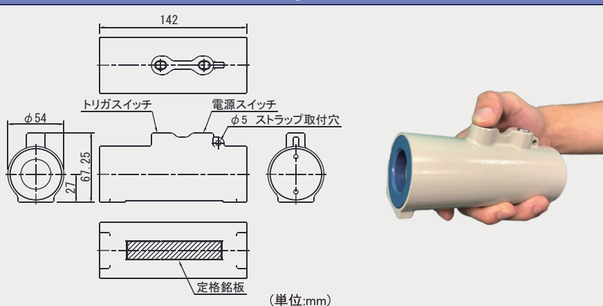
EXSC-QB 外形図
