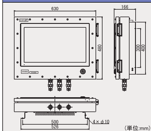
EXPC-6220 外形図
