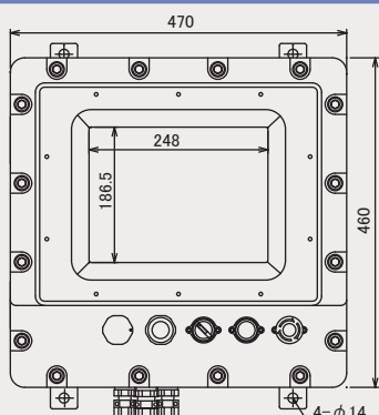
EXGP-3600R 外形図
