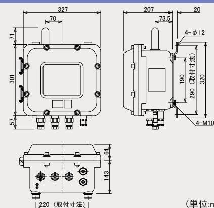
EXWPS-2 外形図
