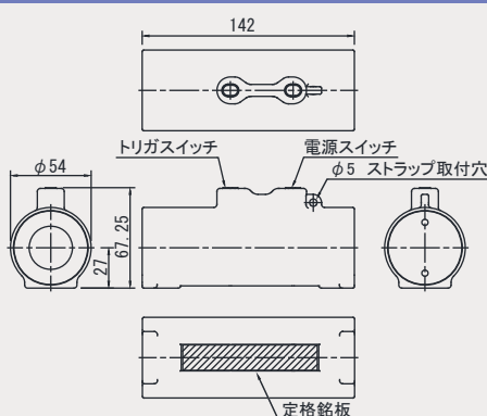
EXSC 外形図
