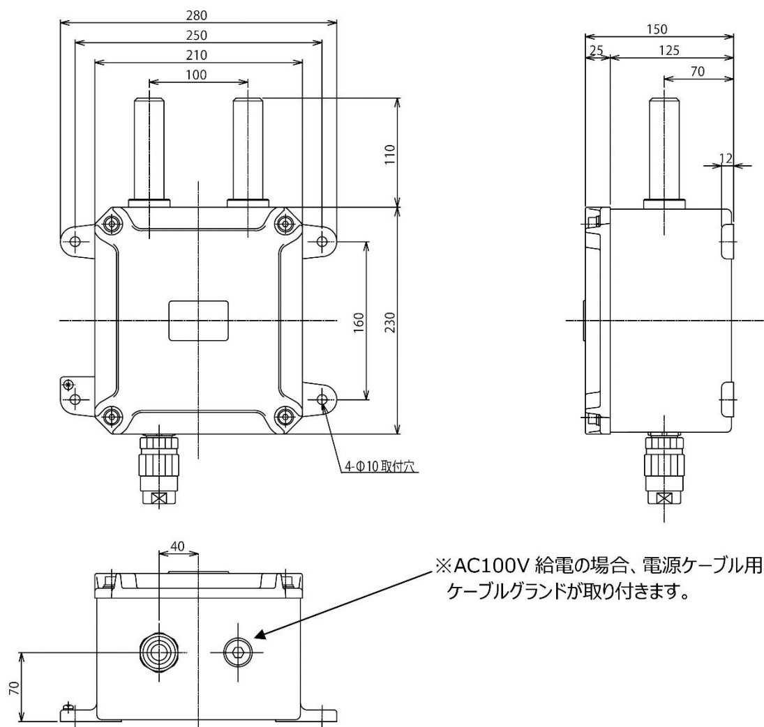
図 2-1 寸法図
