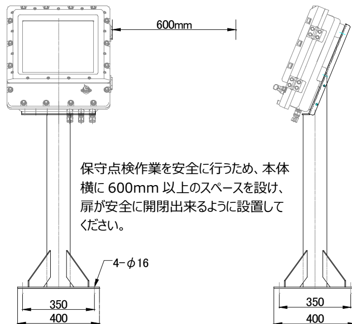
図 4-1 （例）傾斜スタンド EXP-A03740
