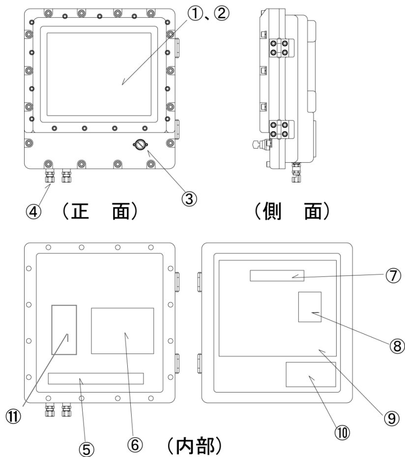
図 3-2 全体図
