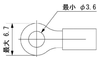
図 4-2 ケーブル端子図
