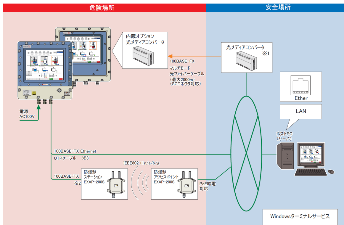
図 2-1 システム構成図
