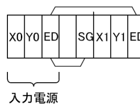
図 4-3 電源端子台
