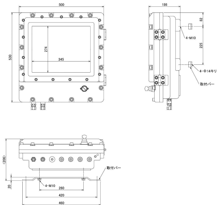
図 3-1 寸法図
