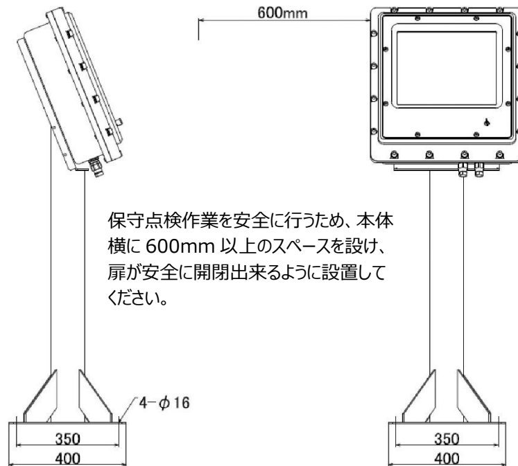
図 4-1 （例）傾斜スタンド EXP-A03740
