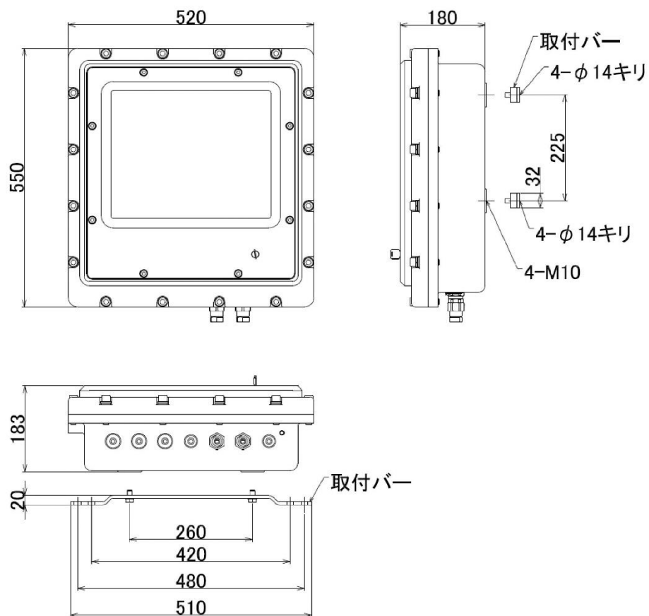
図 3-1 寸法図
