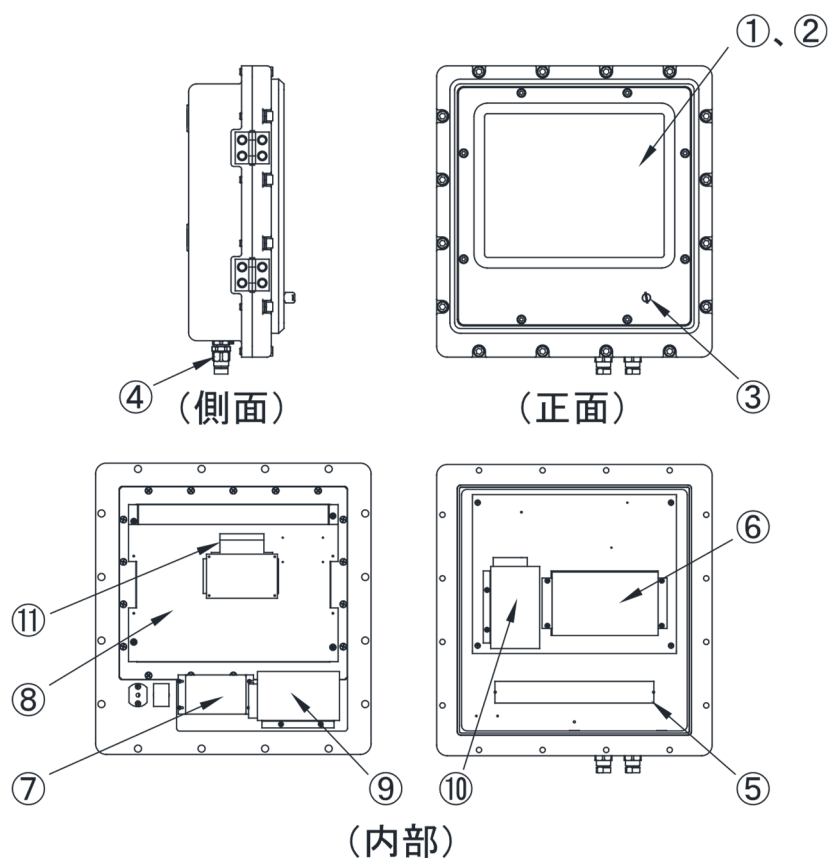
図 3-2 全体図
