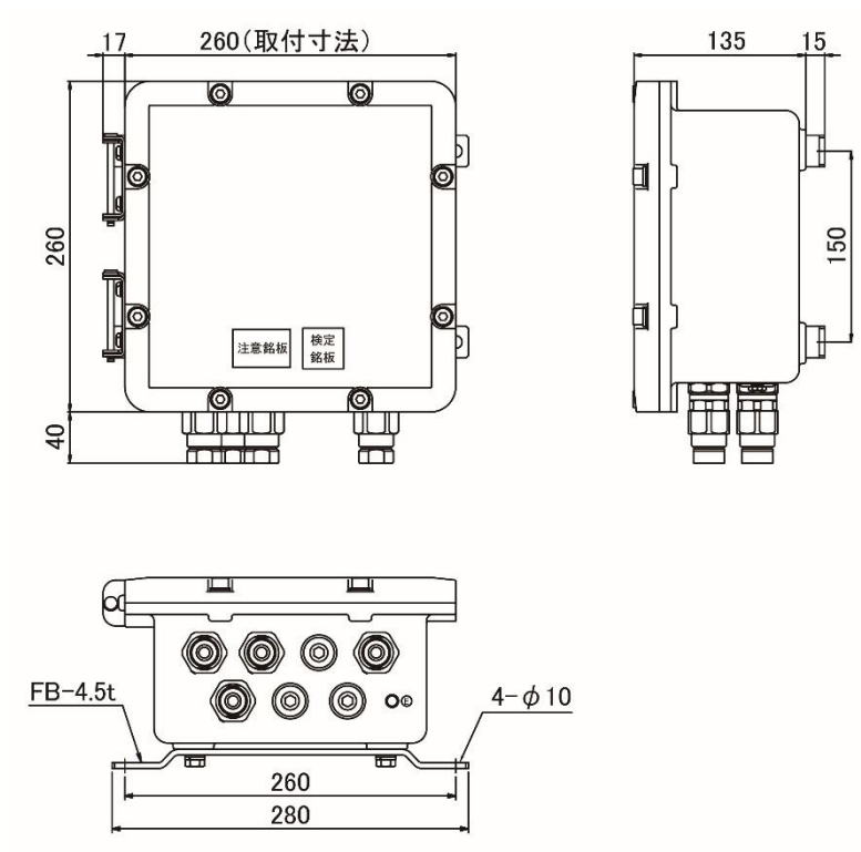
図 2-1 寸法図
