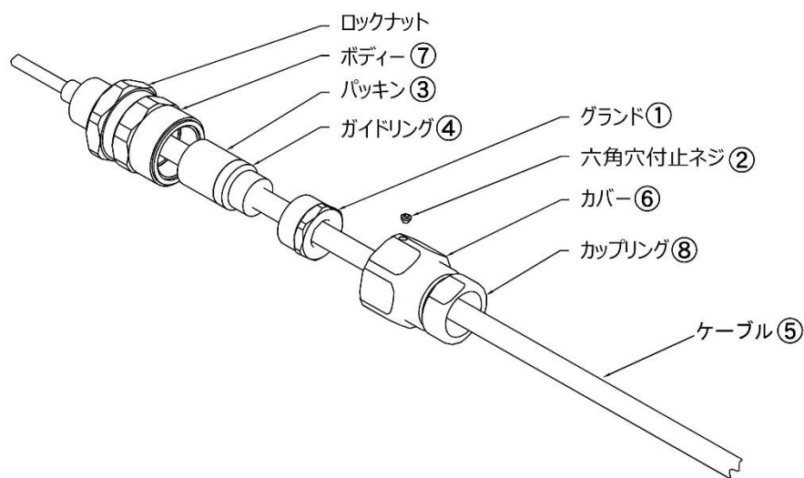
図 3-1 ケーブルグラントでの施工要領
