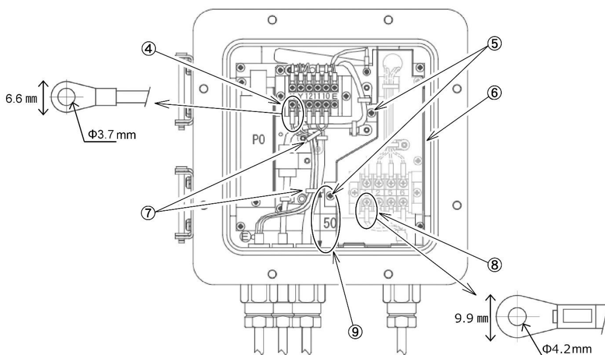
図 3-3 外部導線引込口配置図
