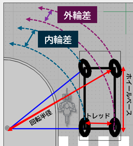
図1. 内輪差・外輪差
