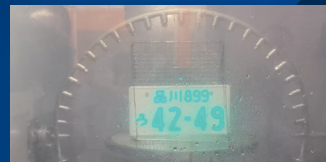
<IPX4K 試験風景>
