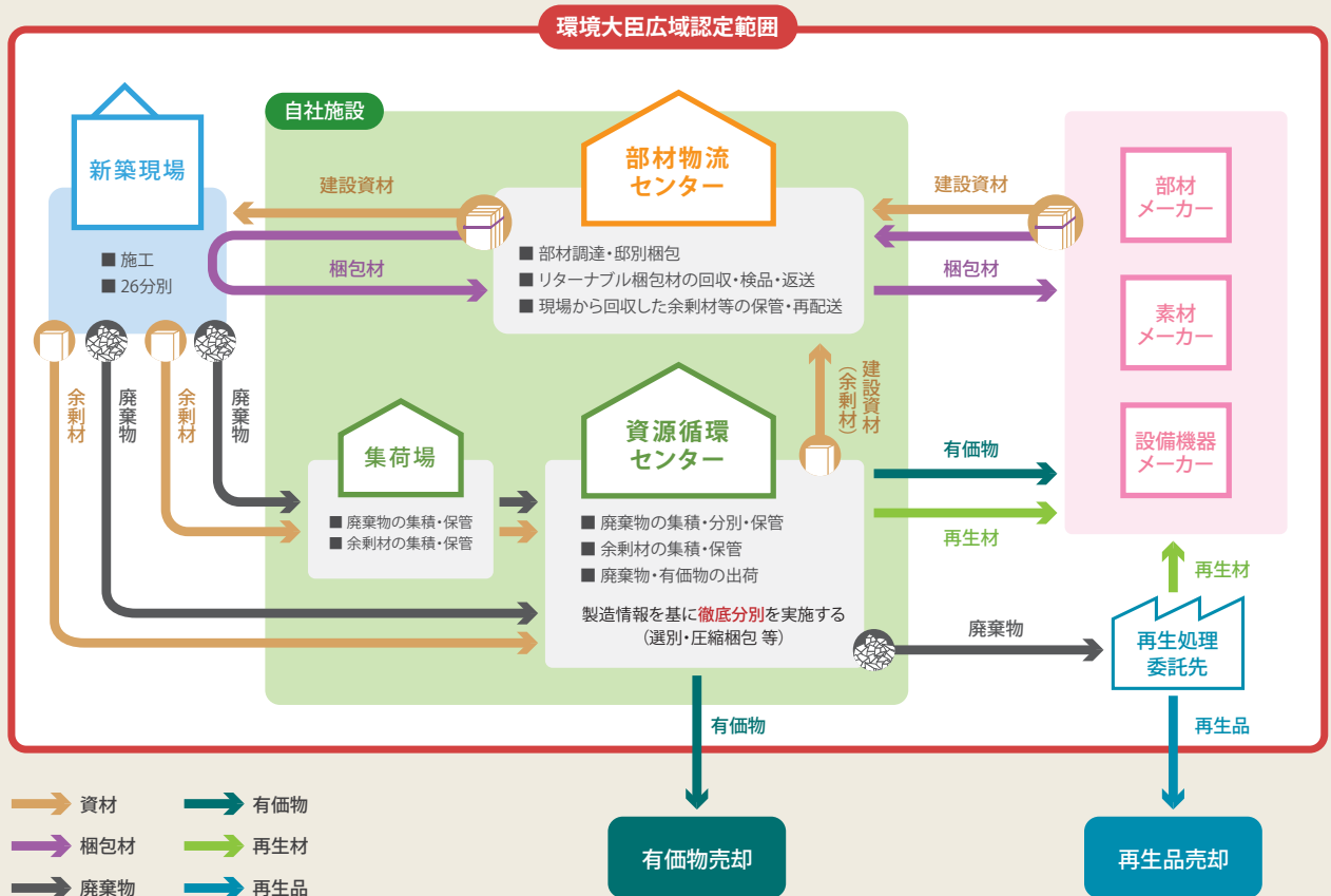
新築ゼロエミッション全体工程図
