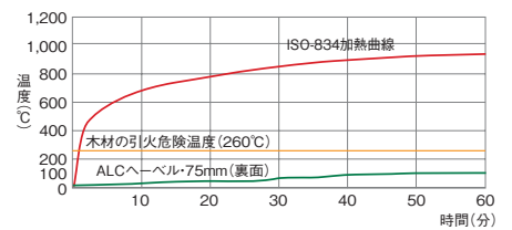
【ISO-834に準じた耐火試験】
