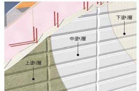
下塗り層：工場塗装 中塗り層・上塗り層：現場塗装
